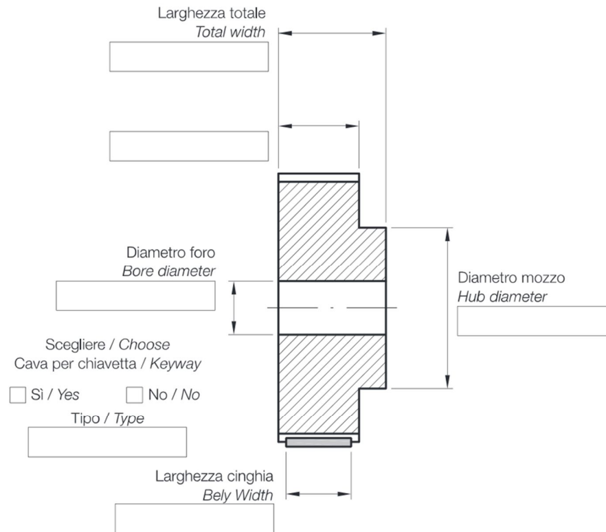
Puleggia con mozzo senza flange - Tipo (B) Pulley with hub, no flanges - Type (B)
