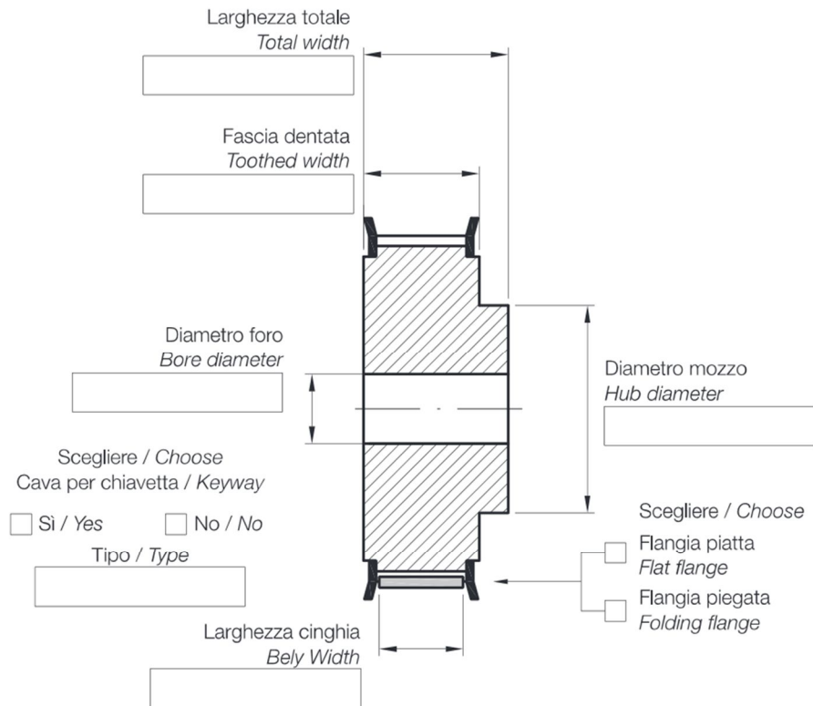
Puleggia con mozzo e flange - Tipo (A) Pulley with hub and flanges - Type (A)
